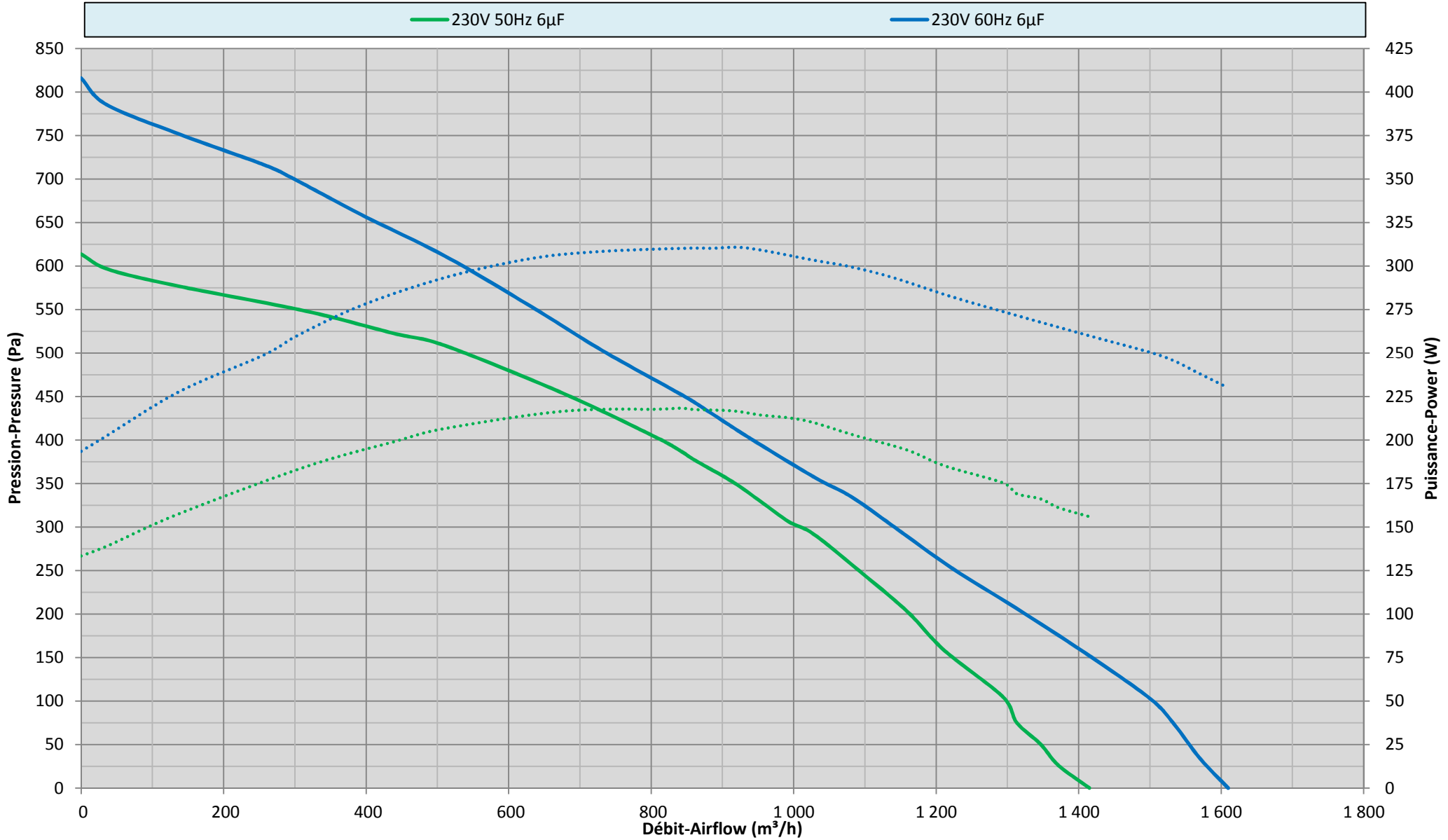
Courbe Débit/Pression-Puissance Airflow/Pressure-Power 2RRE45 250x50R69L1 C=102mm ouie 250R69L
